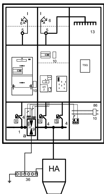
Abb. 1: Spannungsversorgung aus SPD Typ 1
