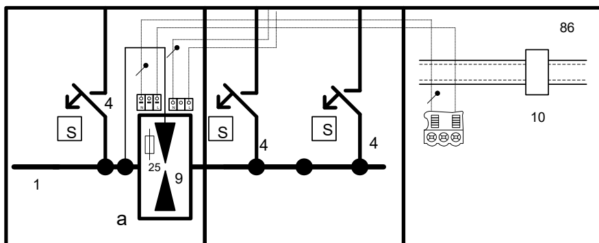
Abb. 4: Netzseitiger Anschlussraum mit Spannungsversorgung aus SPD Typ 1
