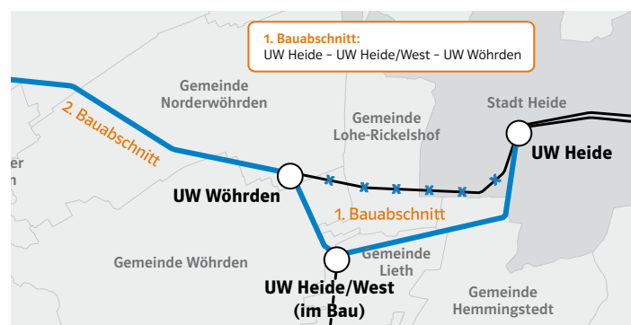
Ausschnitt Trassenverlauf 110-kV-Ersatzneubau Heide - Heide/West - Strübbel
